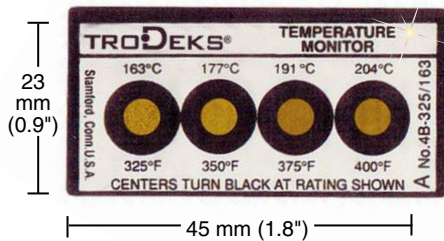
4B-325 shown actual size.
